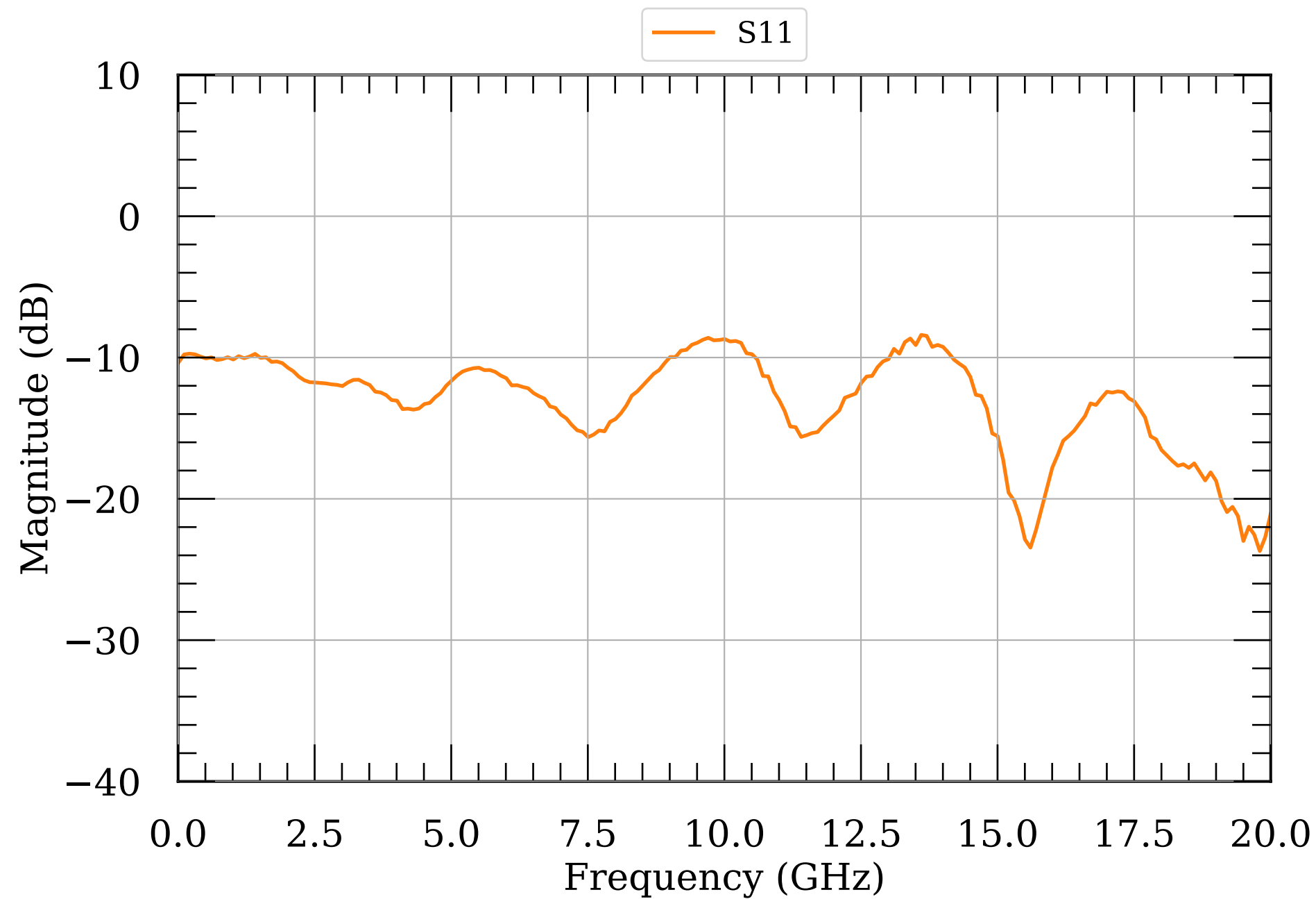
LNA S-params module053V2
